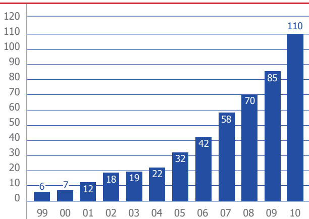
Anzahl der Fotovoltaikanlagen Kundenanlagen und GWG-Anlagen Entwicklung seit 1999
